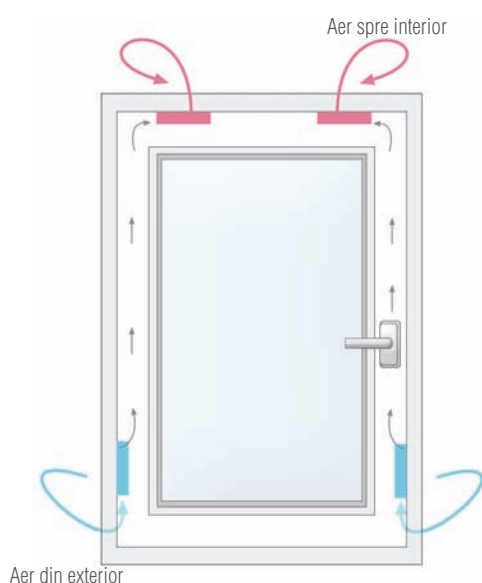
La creșterea presiunii vântului sistemul REHAU AirComfort se închide automat, pe baza principiului lui Bernoulli.
