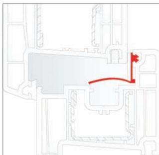
Poziția de aerisire în caz de presiune normală a aerului
