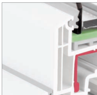
Canat design cu suprafețe suprapuse
